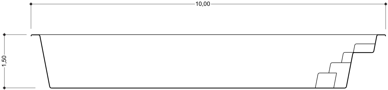
CORTE LONGITUDINAL
