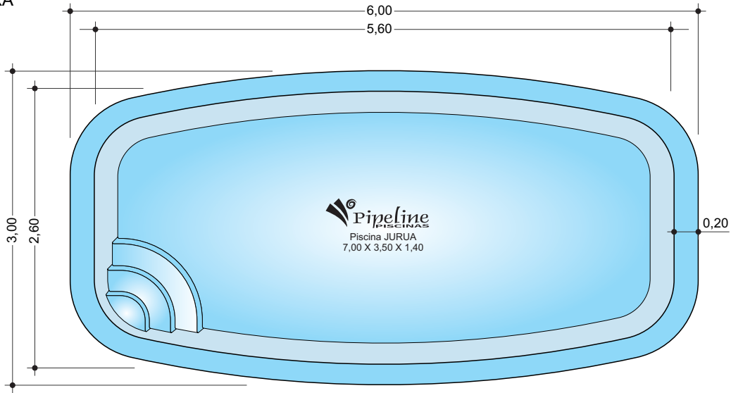
PLANTA BAIXA
