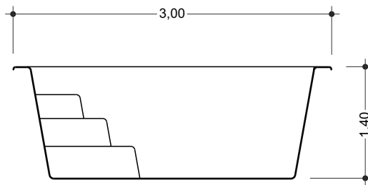
CORTE TRANSVERSAL
