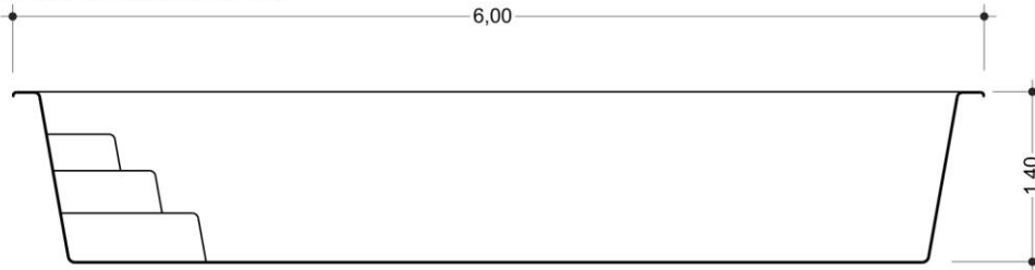
CORTE LONGITUDINAL
