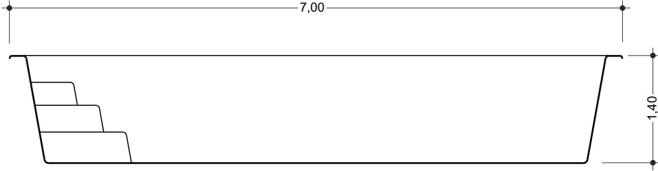
CORTE LONGITUDINAL
