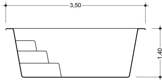
CORTE TRANSVERSAL
