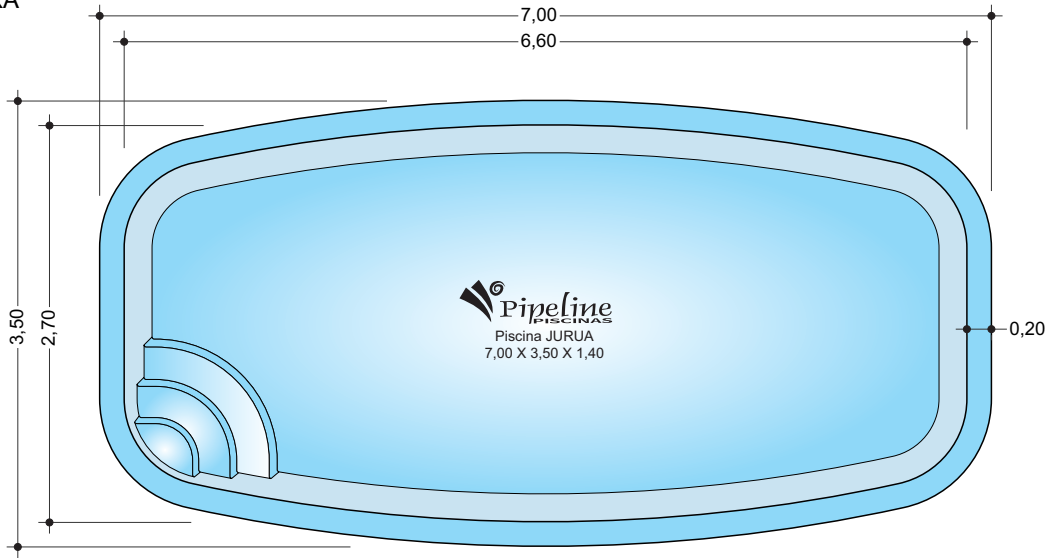
PLANTA BAIXA
